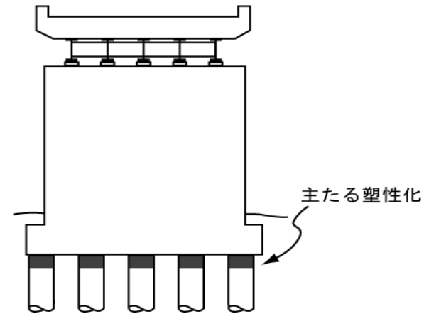
基礎に塑性化を考慮する場合 (壁式橋脚、橋軸直角方向)
