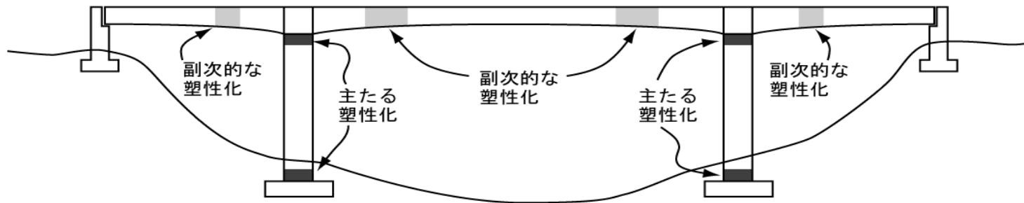
橋脚と上部構造に塑性化を考慮する場合 (ラーメン橋の橋軸方向の場合)
