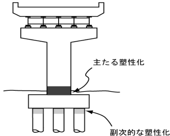
単柱橋脚に塑性化を考慮する場合 (橋軸直角方向)
