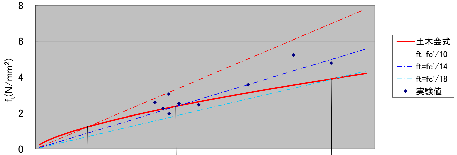
図2 f_t/f_c' と f_c' の関係図
